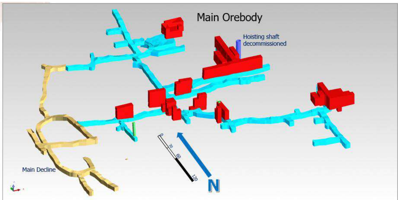
Figure 15.9 Main Orebody, 860 mRL sublevel
