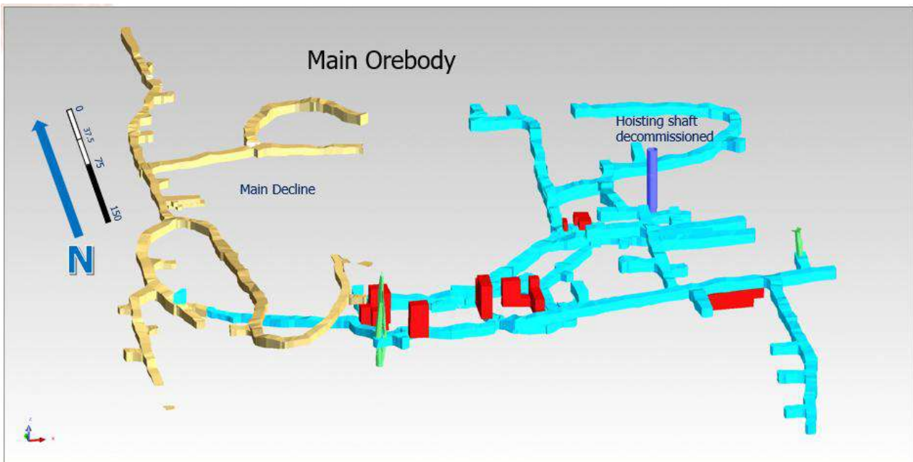
Figure 15.7 Main Orebody, 900 mRL sublevel
