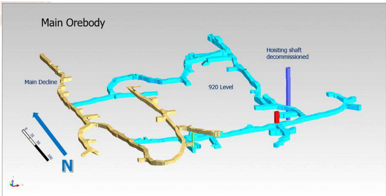
Figure 15.6 Main Orebody, 920 mRL sublevel
