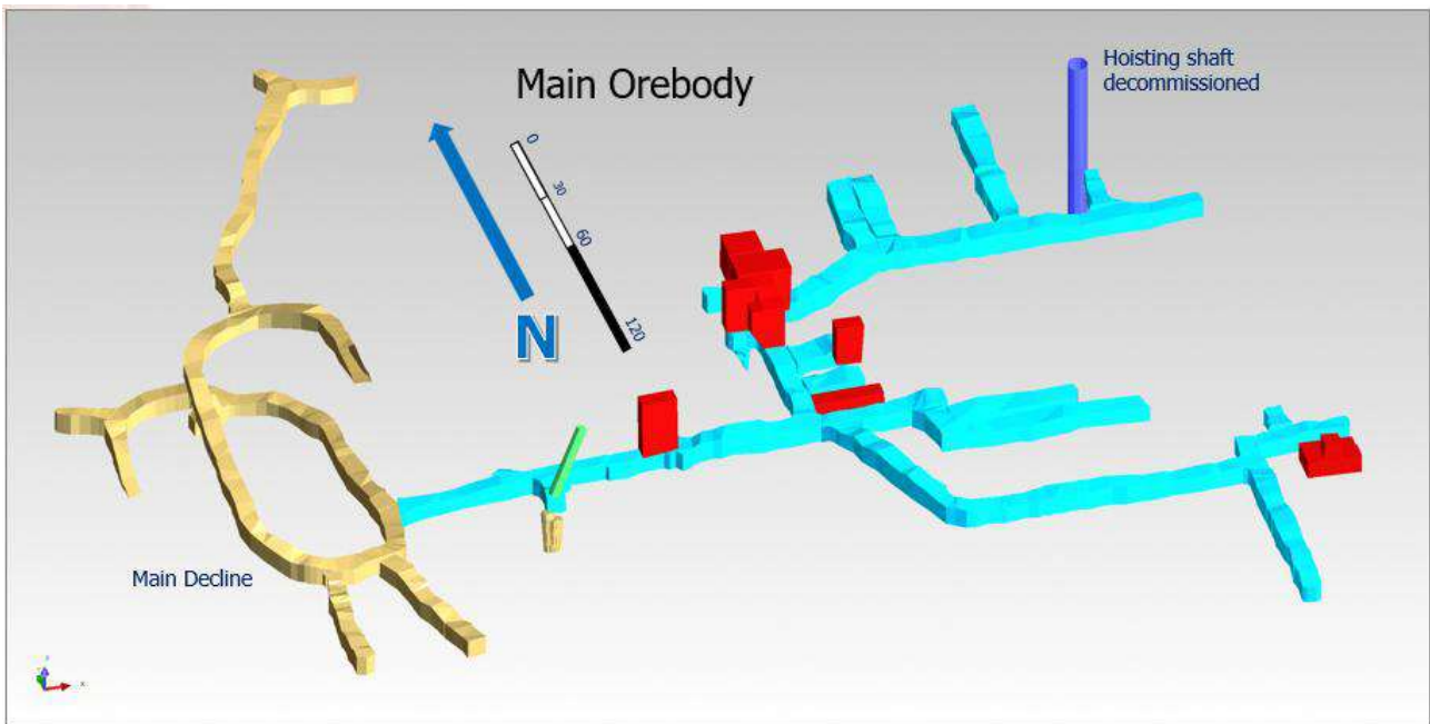
Figure 15.10 Main Orebody, 840 mRL sublevels
